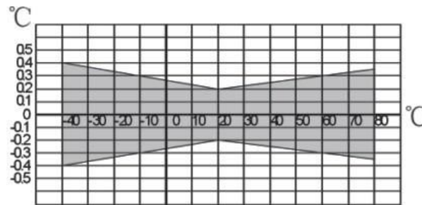
温度误差图
