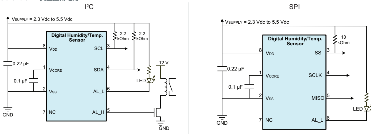
图3: SOIC-8 SMD典型应用电路
