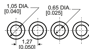
焊盘布局
