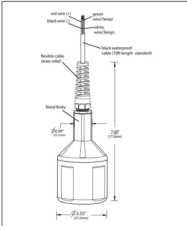
D06400和D07400系列传感器 轮廓图和尺寸
