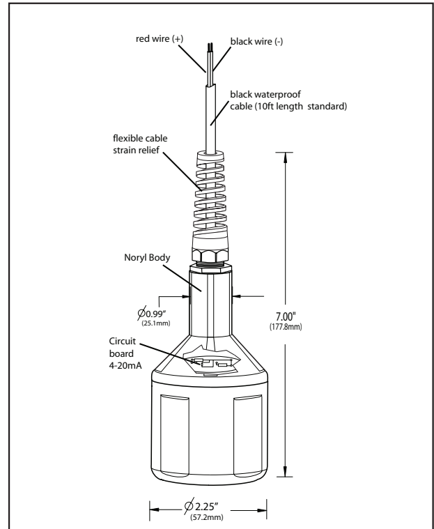
4-20mA 系列传感器 轮廓图和尺寸
