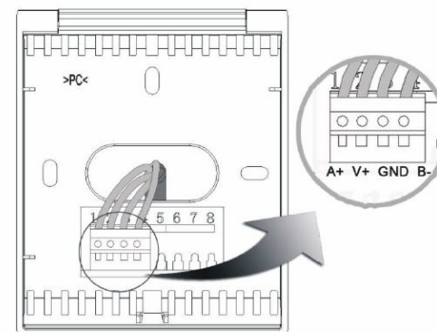
终端接线
