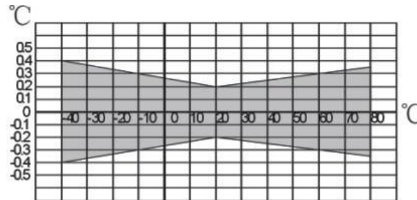
温度误差图
