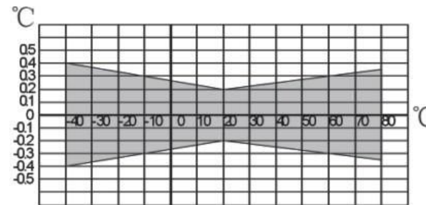
温度误差图
