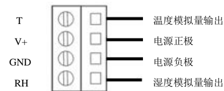
0-10V信号输出接线图
