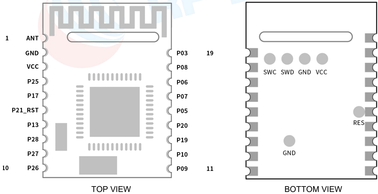
图 3. 引脚图
