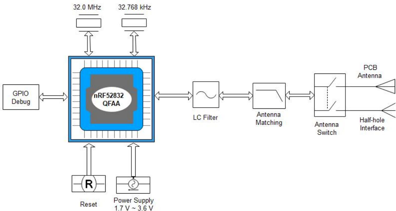
图 1. 原理框图
