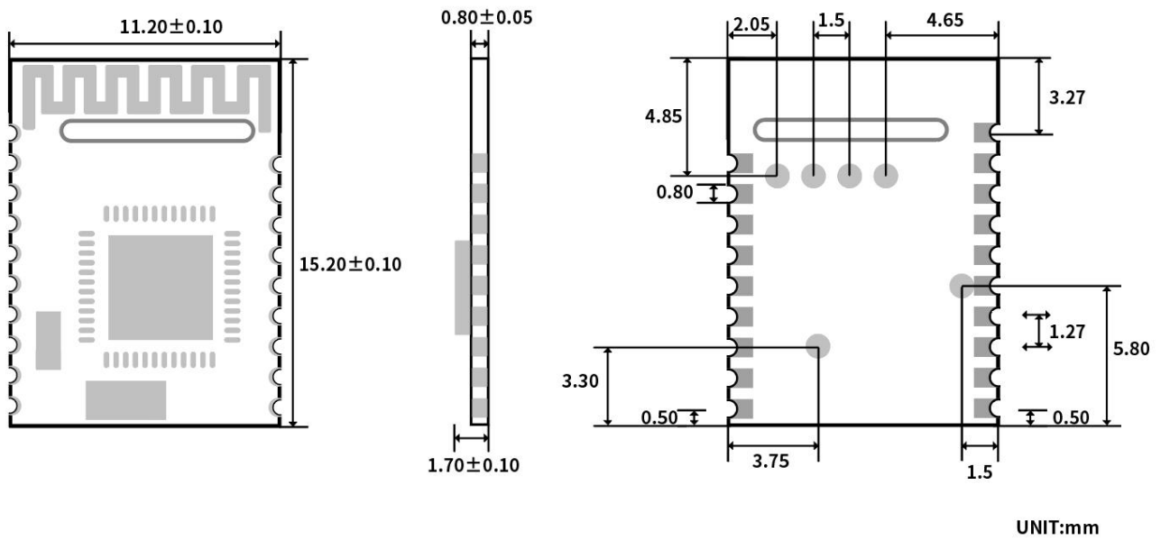
图 2. 尺寸图
